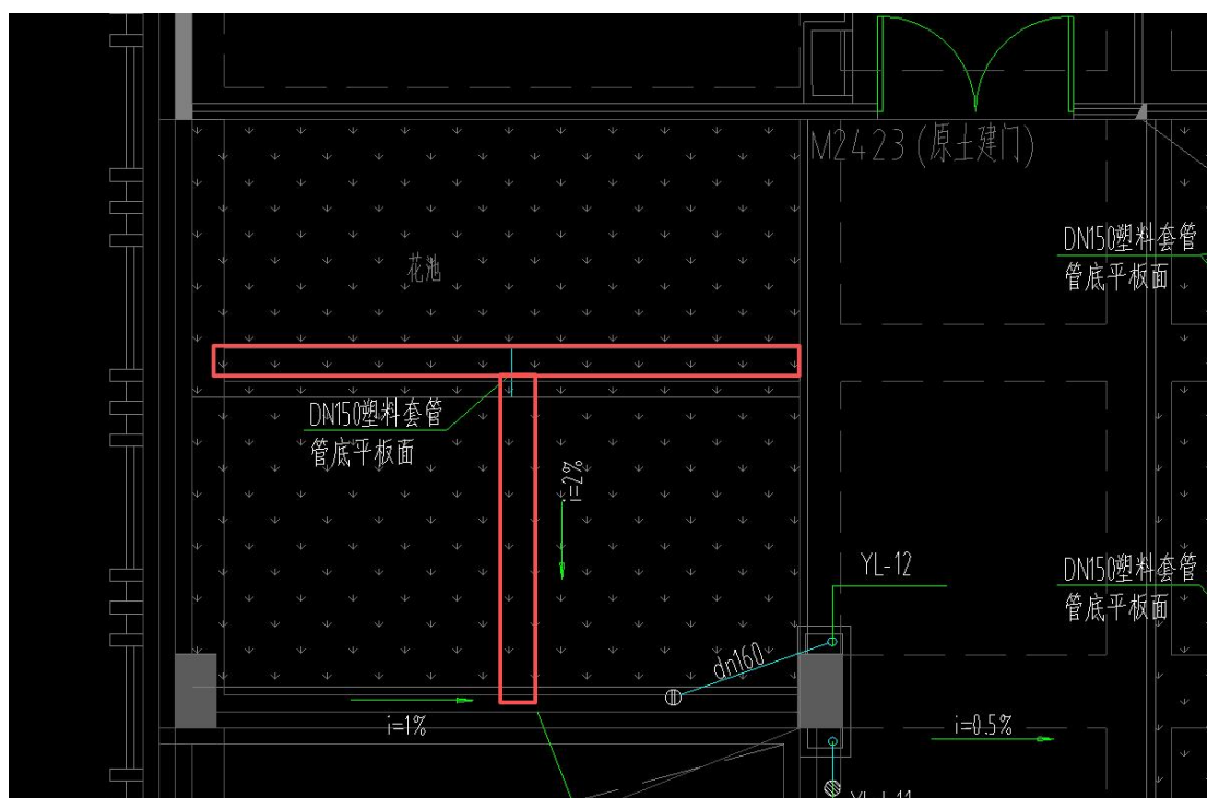
图 三楼西走廊花园绿化带内新建截水沟示意图
