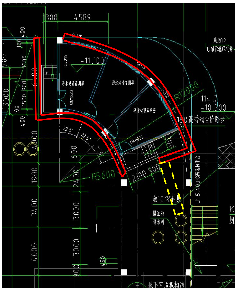
图 急诊科平台缓坡道下方房间外围新建截水沟和暗埋排水管示意图
