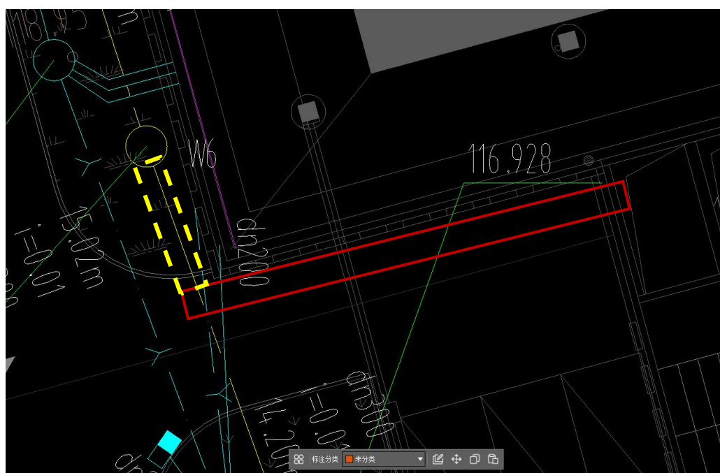
图 负一楼停车场入口处新建截水沟和暗埋排水管示意图
